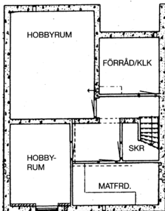
2 rok 51 m 2 Hillersjövägen, Källarplan
